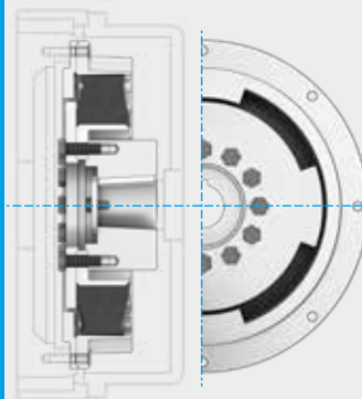
Type AC...F2 DS
